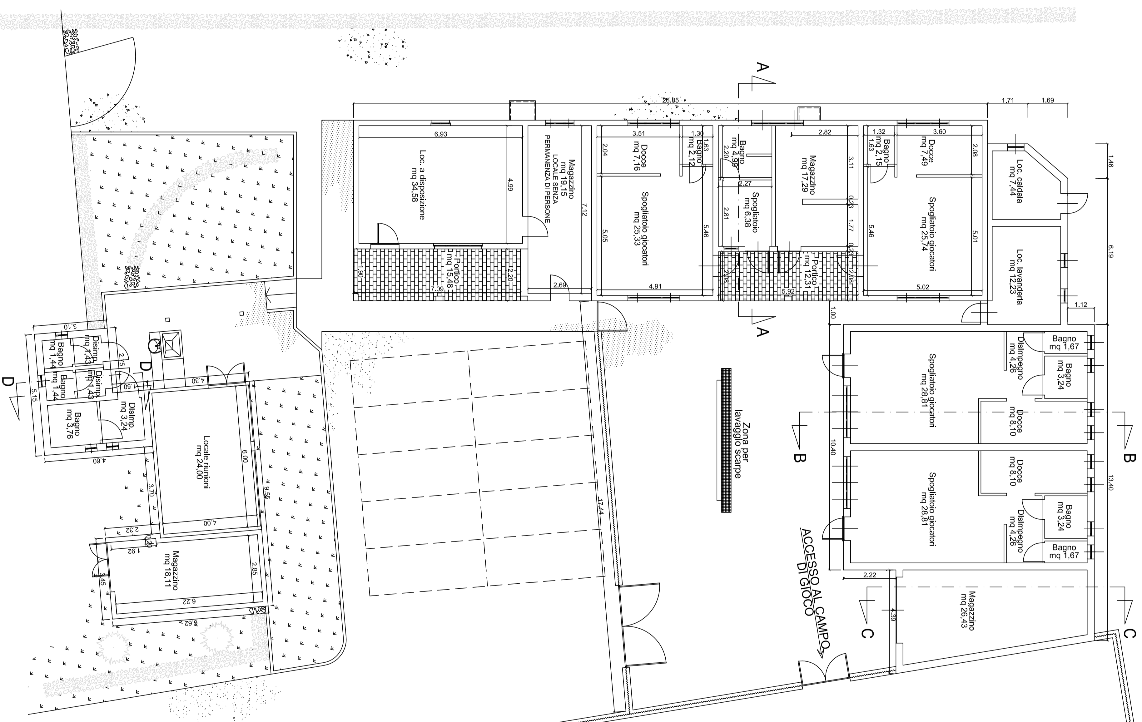
Pianta piano terra: progetto
