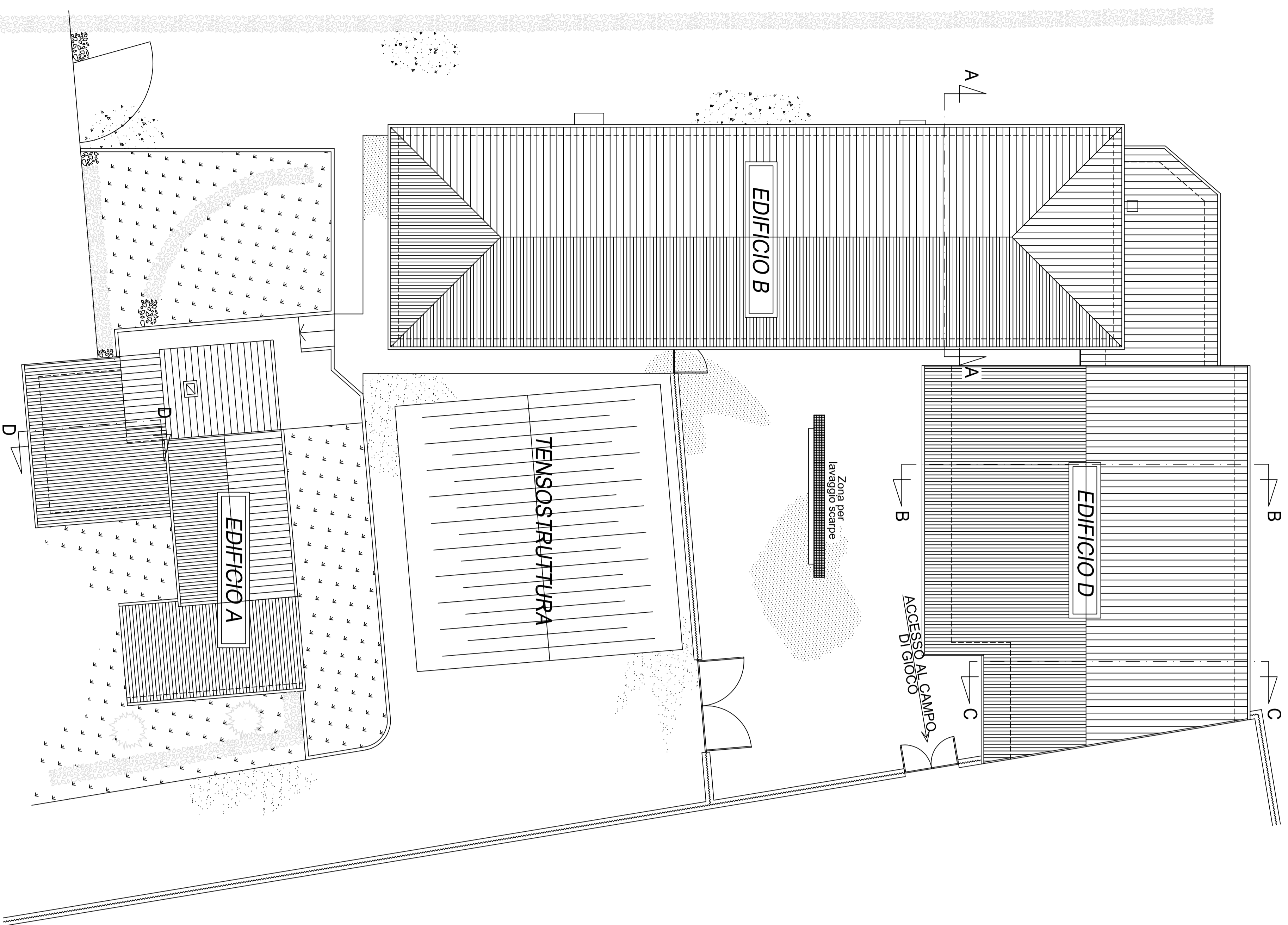
Pianta copertura: progetto
