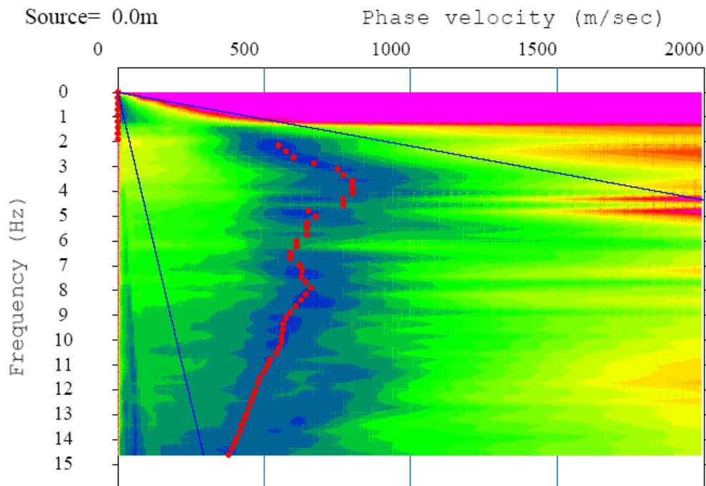
Curva di dispersione REMI
