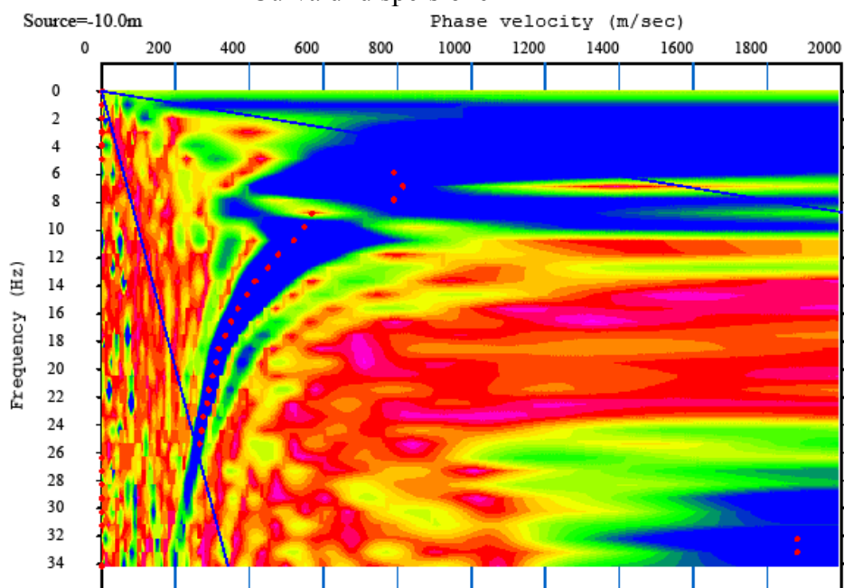
Curva di dispersione MASW
