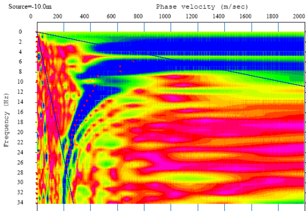
Curva di dispersione MASW
